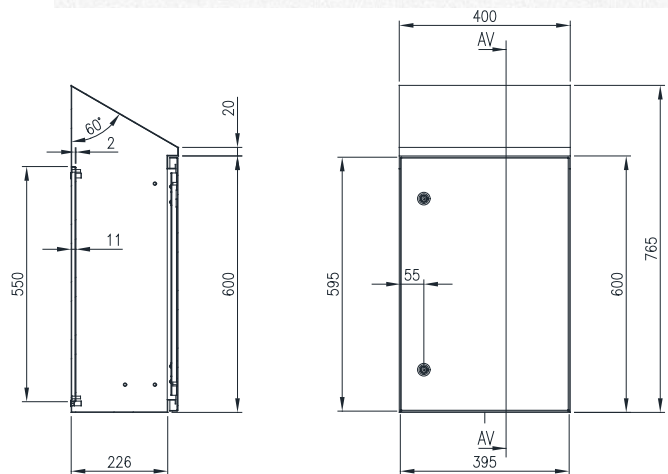
SECTION AV-AV
