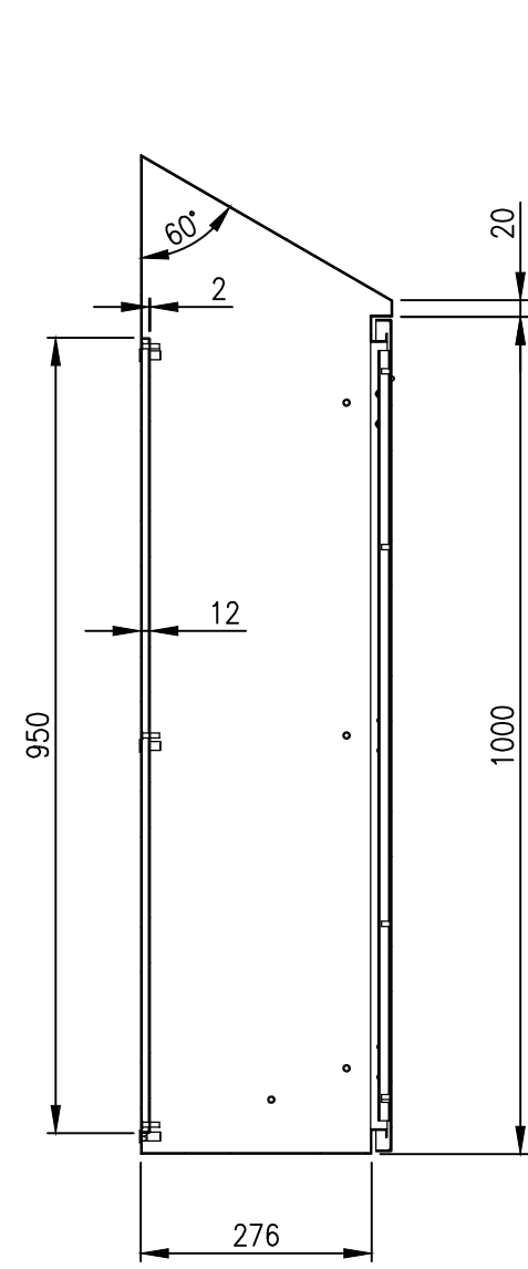
SECTION AV-AV
