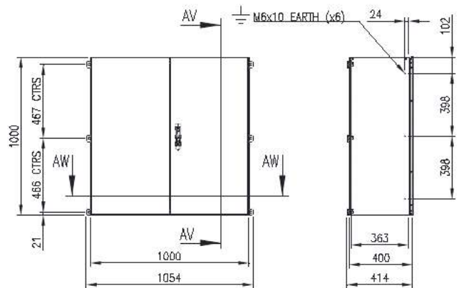
SECTION AV-AV
