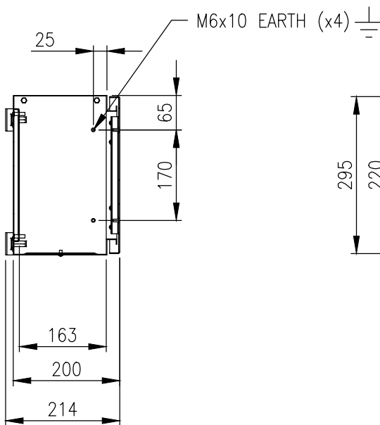
SECTION AV-AV
